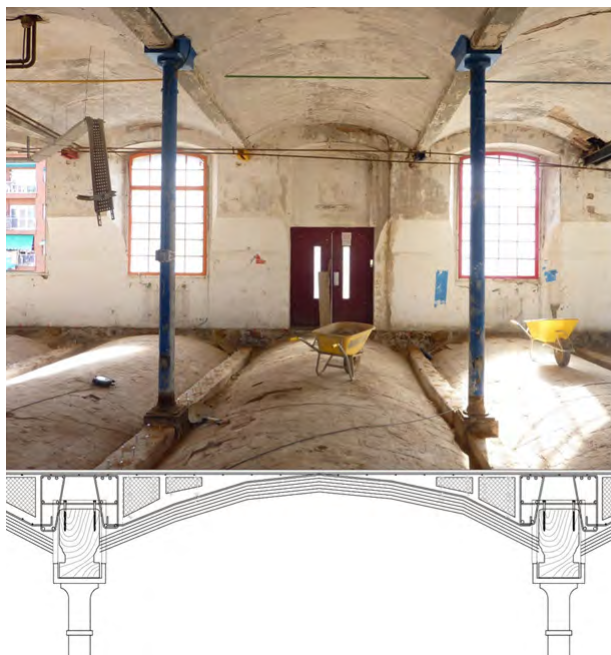
Imagen 5. La estructura. Plano sección de proyecto ejecutivo.
